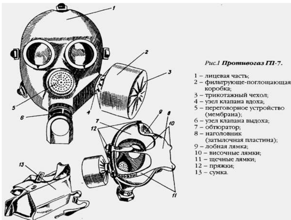
Рисунок 2- Противогаз ГП-7
