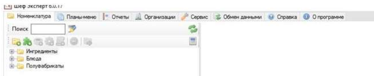
Рисунок 1 – Интерфейс программы
