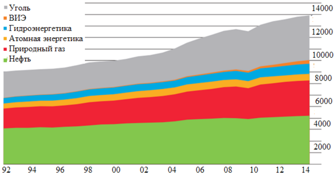
Рисунок 1 – Мировое потребление энергоресурсов, млн. TOE (ton of oil equivalent) [16]
