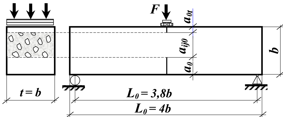
Рис. 1. Образец типа 1 по ГОСТ 29167-91 для испытания на изгиб для определения характеристик трещиностойкости при равновесных испытаниях
