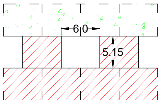
Рисунок 2.3 – Параметры выемочных заходок на руднике «Айхал»
